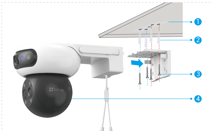
Afb. 1 Plafondmontage
