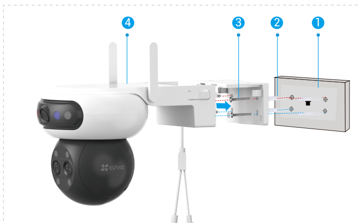
Afb. 2 Muurmontage
